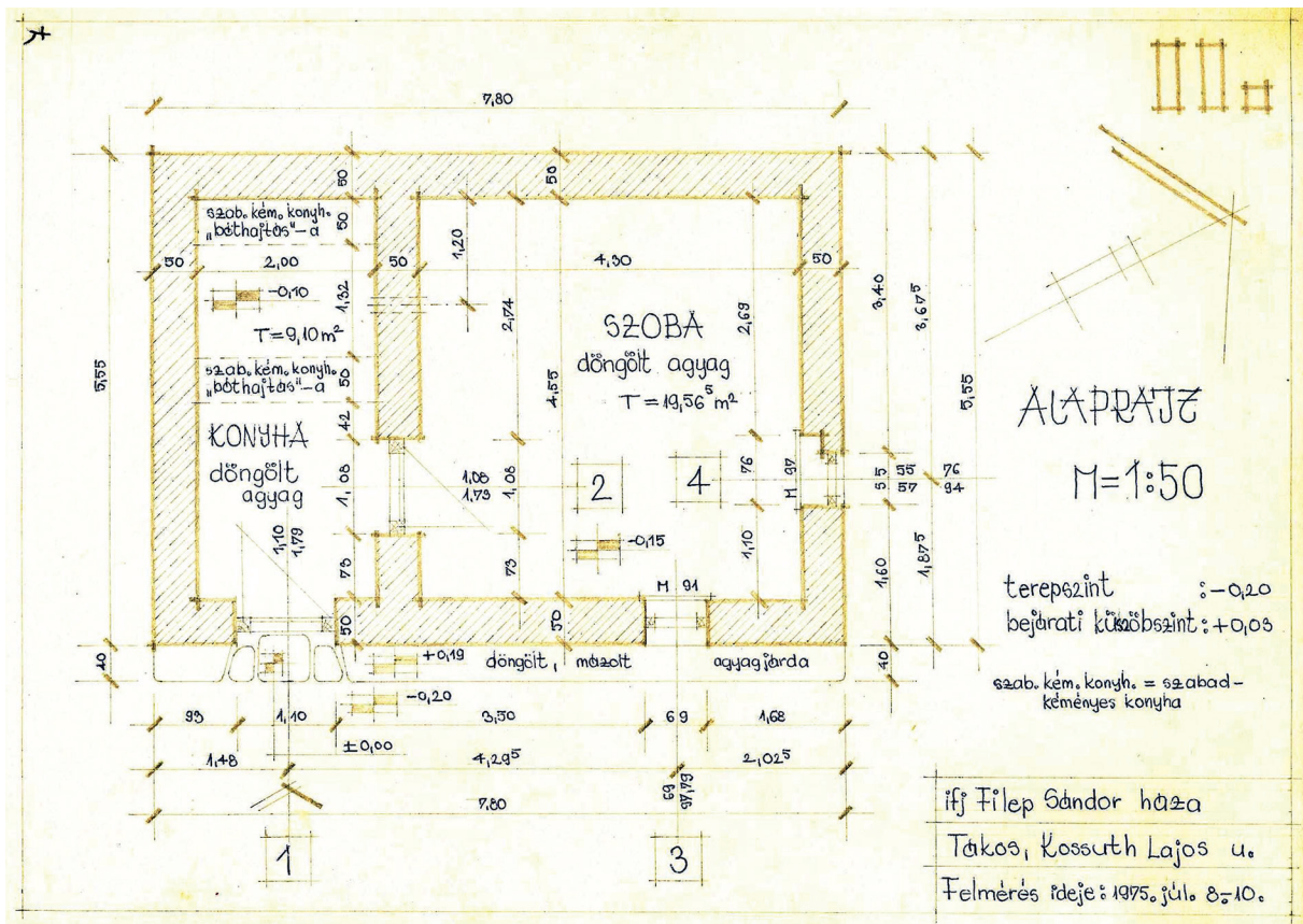
Parasztház alaprajza / Ground plan of a peasant house
